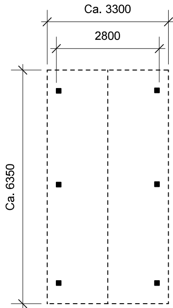
Plantegning
