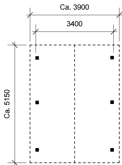
Plantegning
