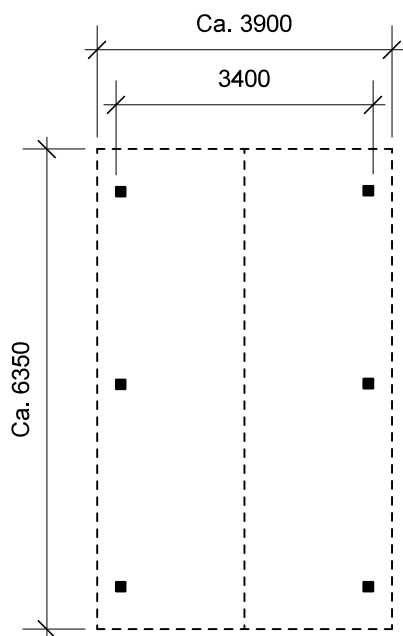
Plantegning
