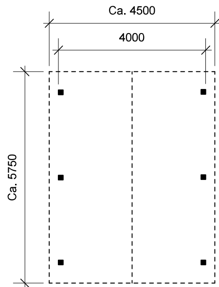
Plantegning
