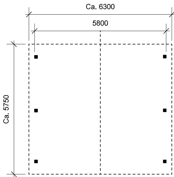
Plantegning
