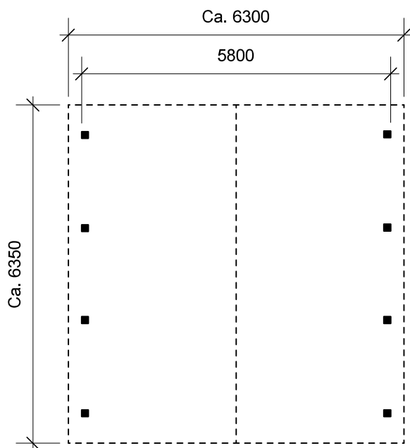
Plantegning
