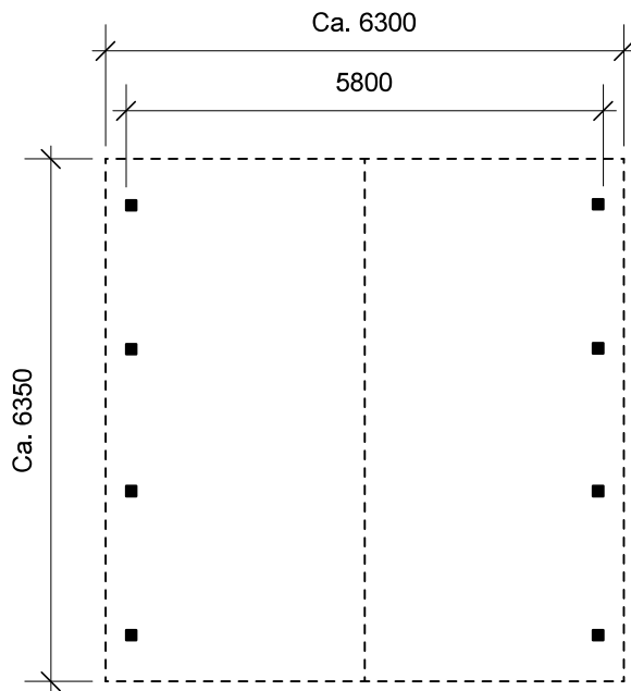
Plantegning
