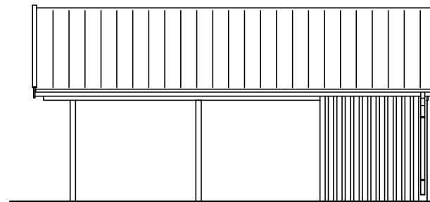
Facade - venstre
