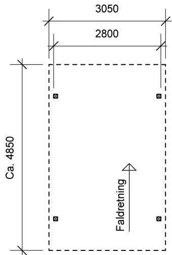
Plantegning
