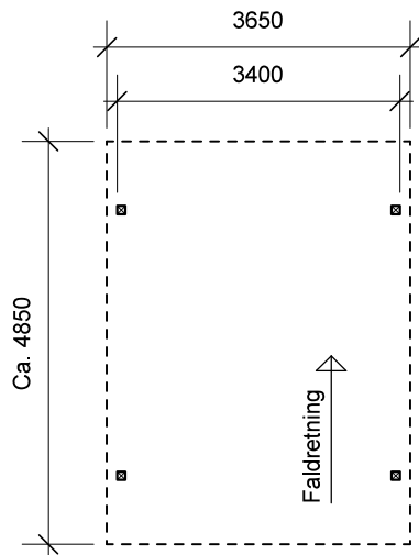
Plantegning
