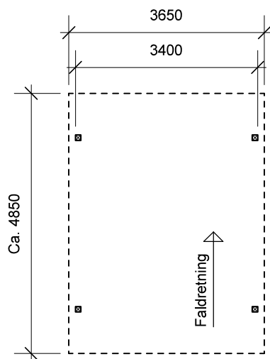
Plantegning
