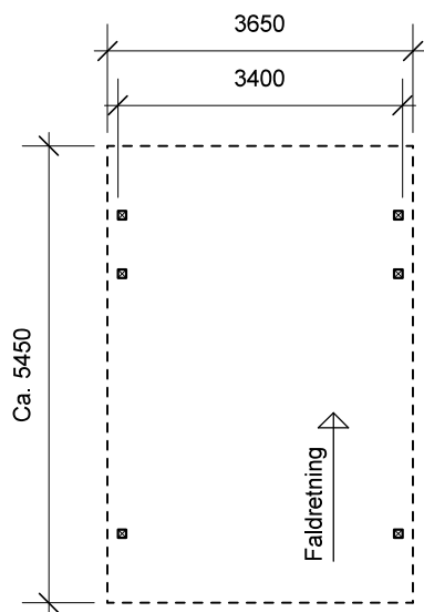
Plantegning
