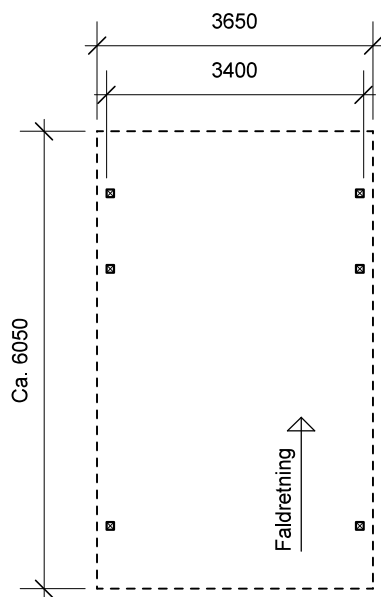
Plantegning
