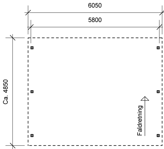
Plantegning
