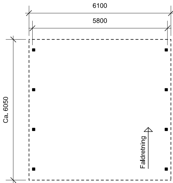
Plantegning
