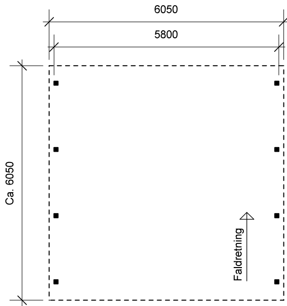
Plantegning
