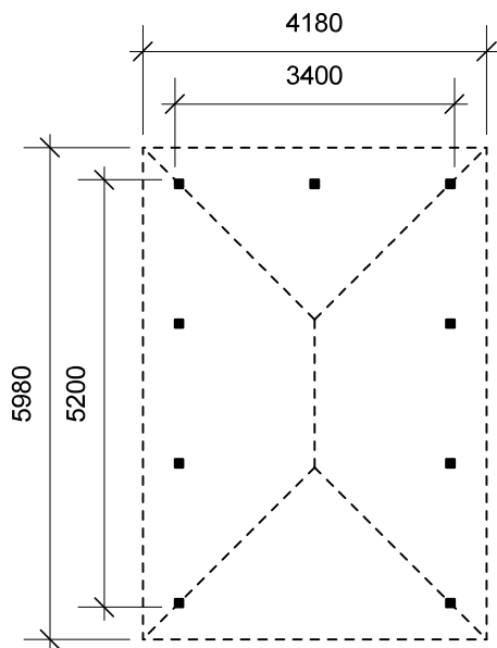
Plantegning
