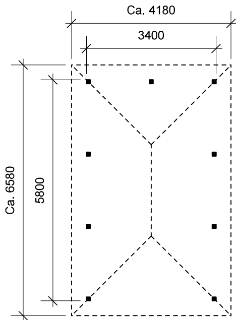
Plantegning
