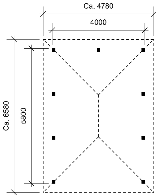
Plantegning
