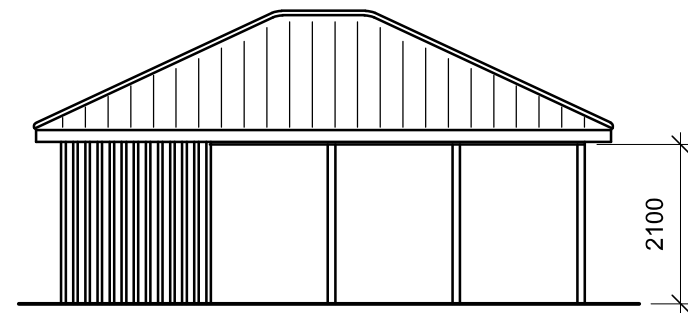
Facade - venstre
