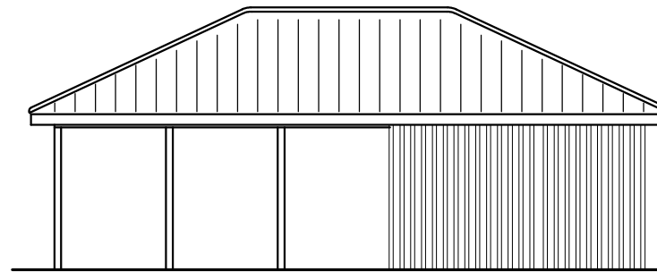
Facade - højre
