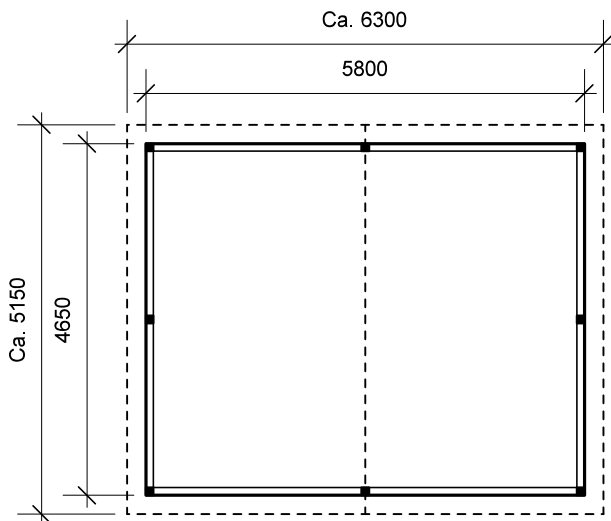
Plantegning
