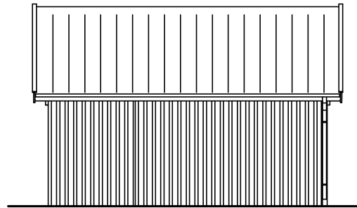
Facade - venstre
