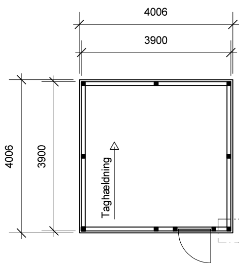
Plantegning
