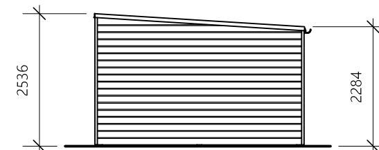
Facade - højre
