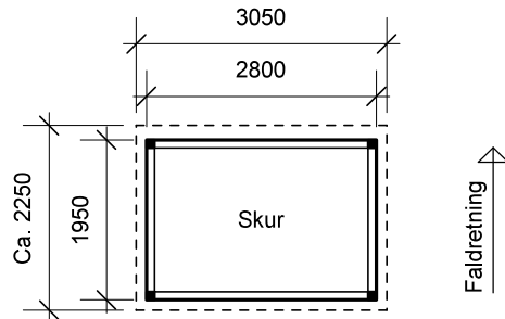
Plantegning
