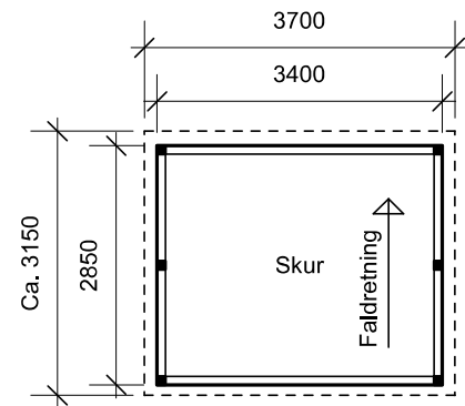
Plantegning
