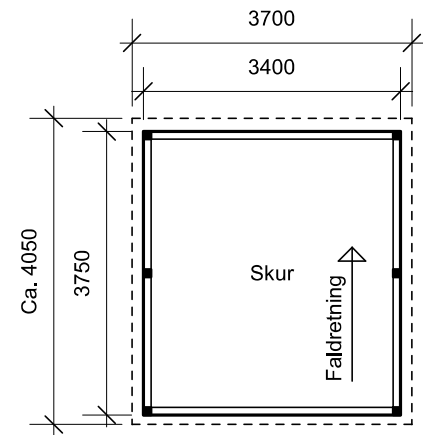
Plantegning
