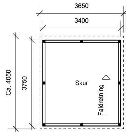
Plantegning
