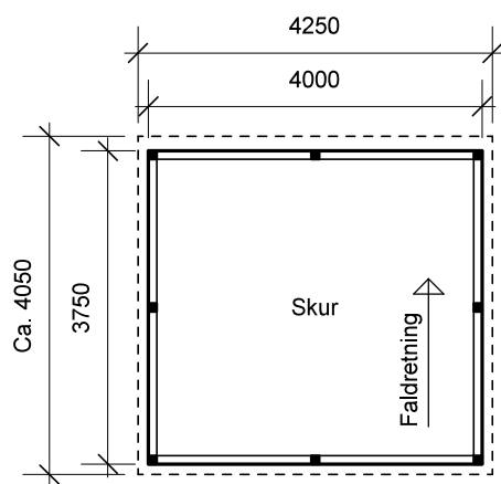
Plantegning
