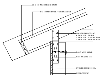
SNIT 1:50
