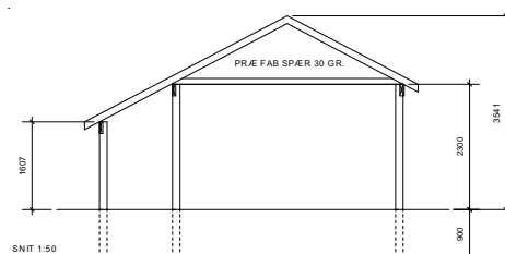
SNIT 1:50
