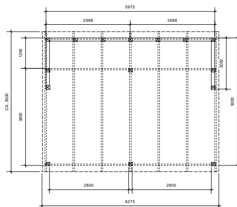
PLAN 1:50
